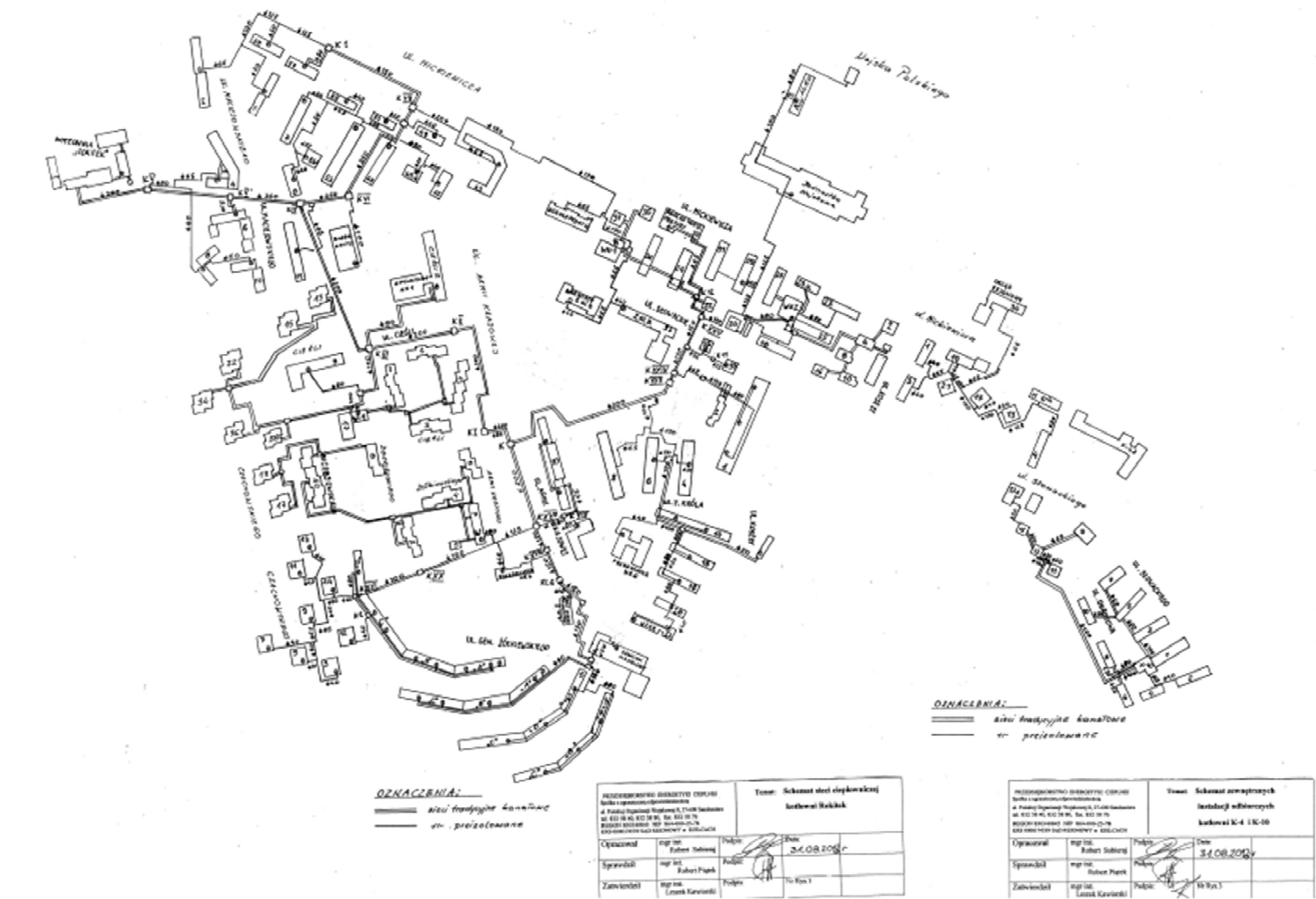
Załącznik 1 Schemat sieci ciepłowniczej ROKITEK
